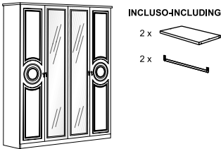
4 door wardrobe Armoire 4 portes W. 176,5 D. 53 H. 219 Vol. 0,41 mc - Box 8 - Kg 168,10
