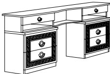
Vanity dresser Coiffeuse W. 173 D. 37,5 H. 75 Vol. 0,52 mc - Box 3 - Kg 68,90
